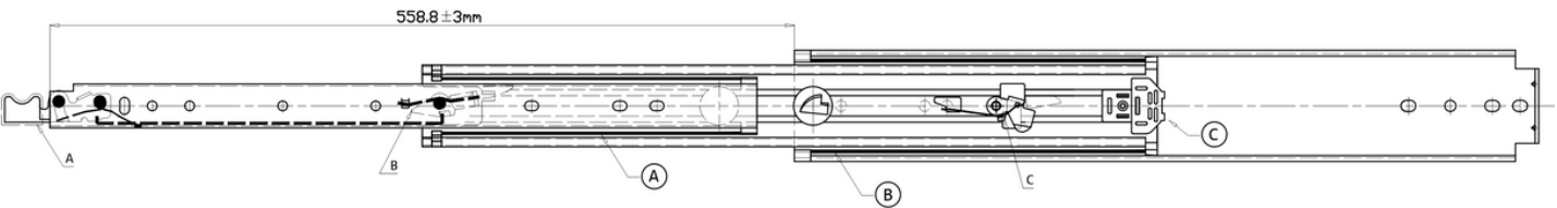
Długość ekstrakcji (wysuwu)
