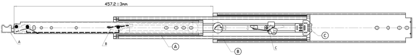
Długość ekstrakcji (wysuwu)
