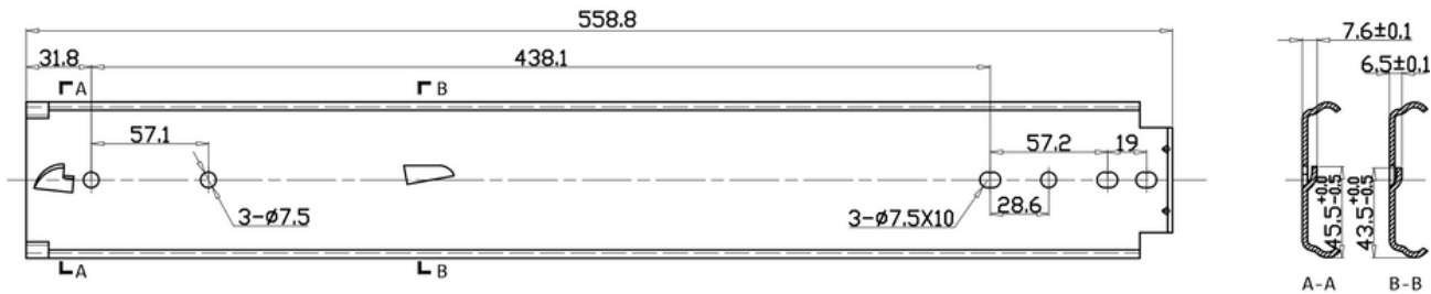
Długość szyny środkowej
