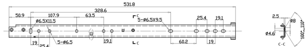
Długość szyny wewnętrznej
